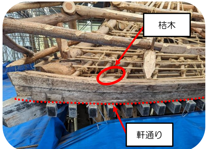
②桔木を入れたことで軒通りがよくなりました。破損が激しい下地の丸太は新材に交換しました。
