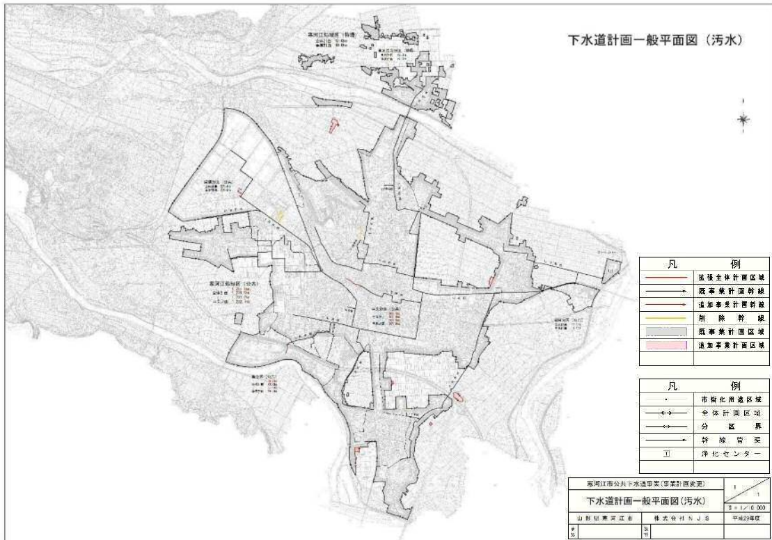
[図-1] 下水道計画一般図(汚水)
