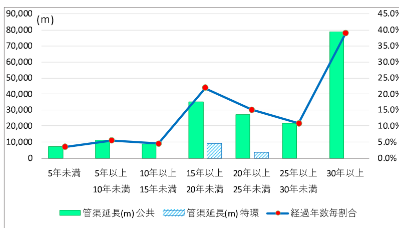
[図-7] 汚水管経過年数毎延長割合比較
