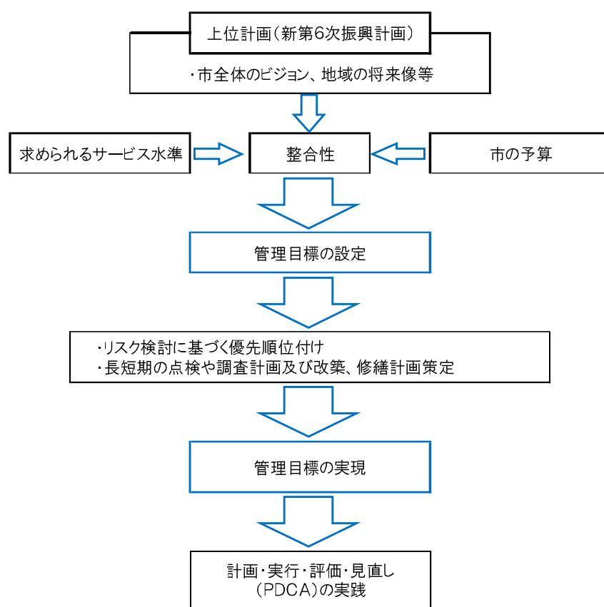
[図-23] ストックマネジメントのフロー
