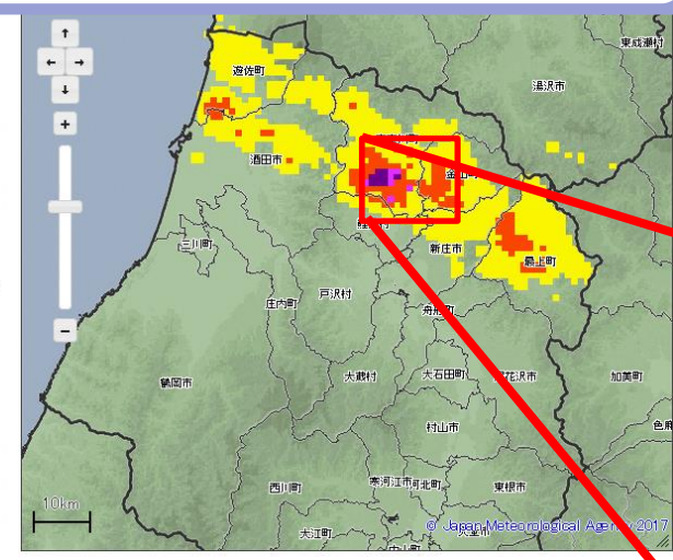
大雨警報(土砂災害)の危険度分布 (土砂災害警戒判定メッシュ情報)
