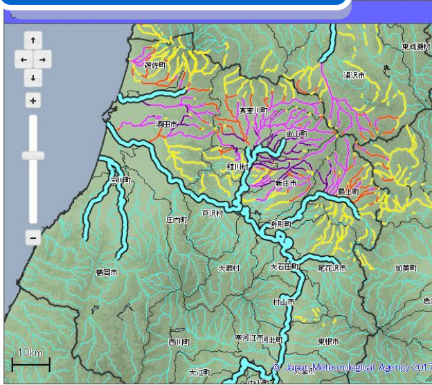
洪水警報の危険度分布
