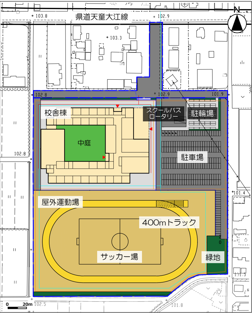
新中学校施設整備の基本計画案 校舎棟を北、屋外運動場を南に配置する形態
