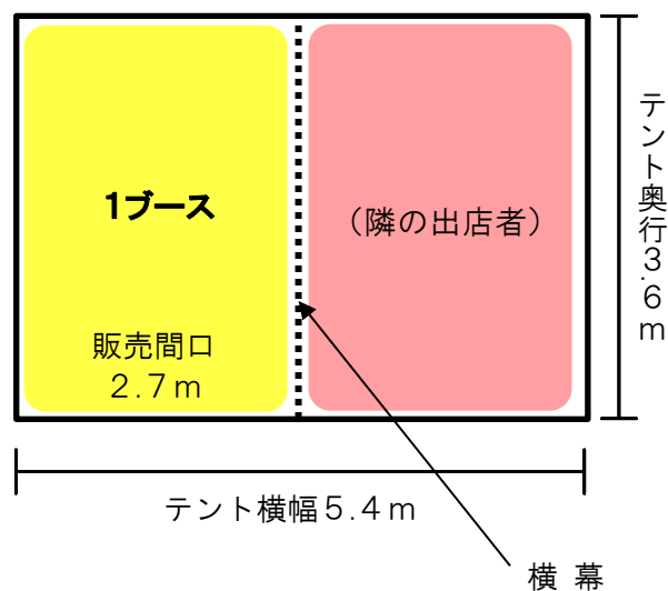
◎平面図
