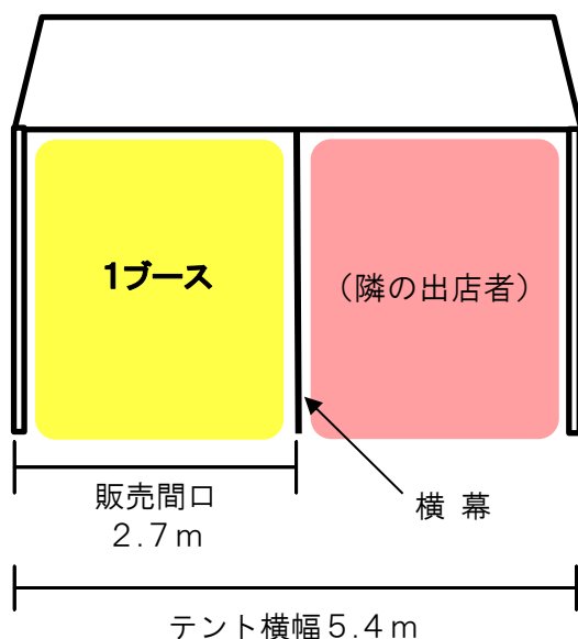
◎立面図
